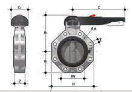
FKOV/LM LUG ISO-DIN Vanne à papillon à commande manuelle, version Lug ISO-DIN
