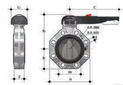
FKOV/LM Vanne à papillon à commande manuelle
