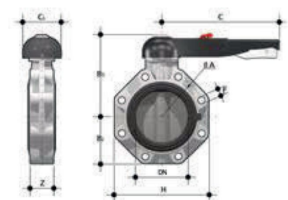
FKOV/LM LUG ANSI Vanne à papillon à commande manuelle, version Lug ANSI
